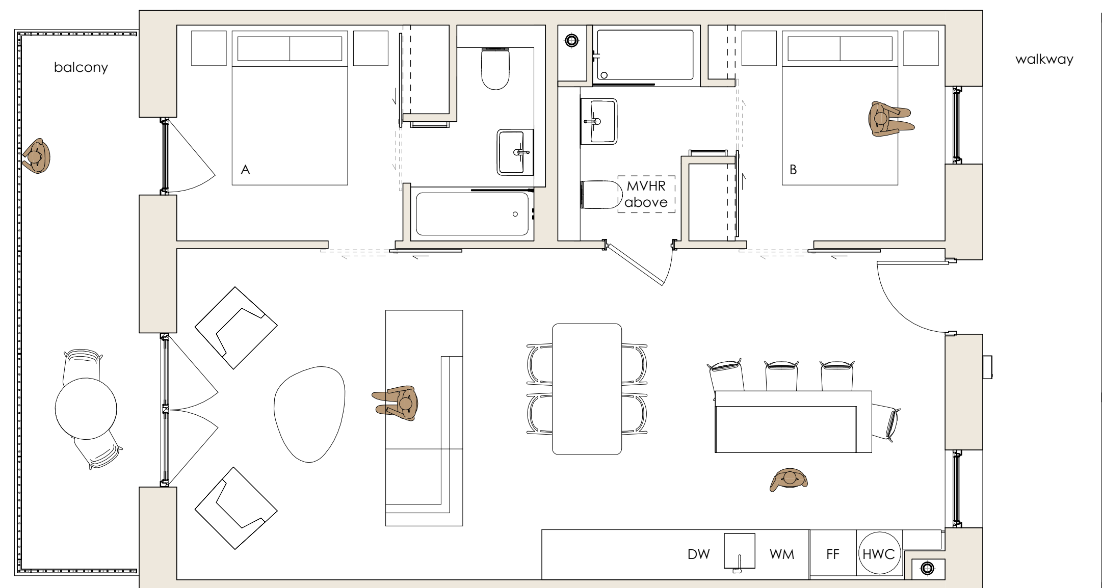
PLAN 1:50
